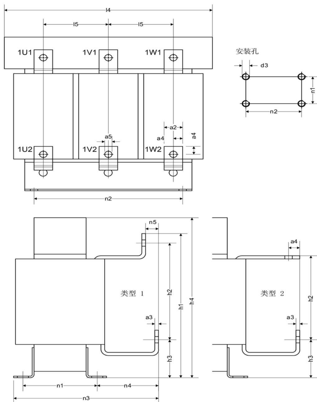
图 3-1 电机电抗器的外形尺寸图
